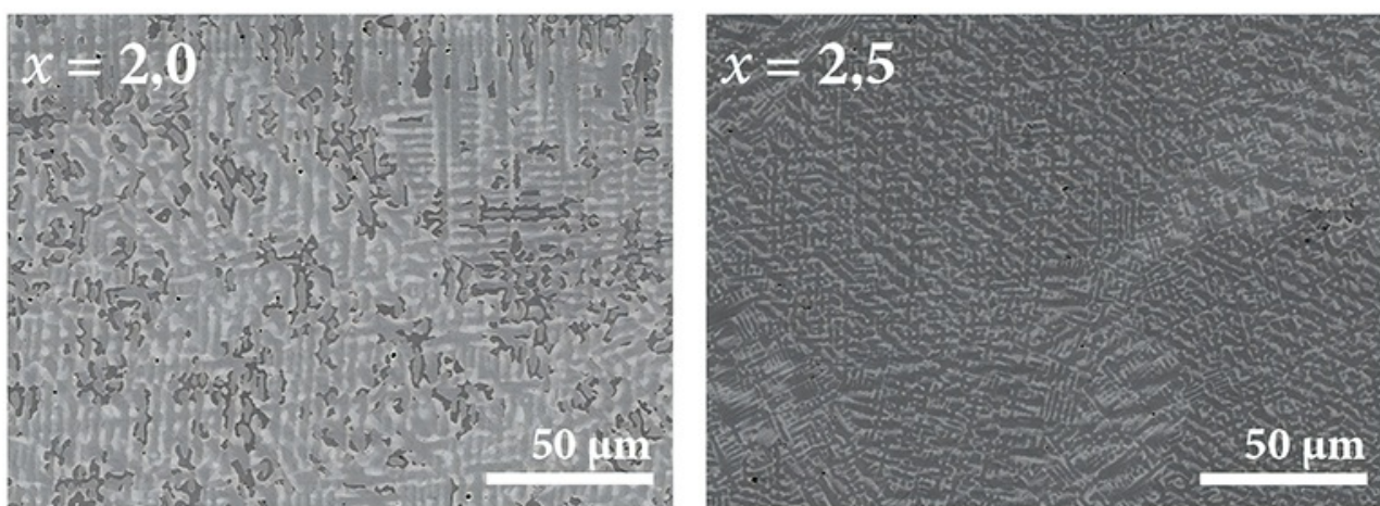
Slika 3: Slike vzorcev \text{AlCoFeNiCu}_{2,0} in \text{AlCoFeNiCu}_{2,5} , posneti z vrstičnim elektronskim mikroskopom (angl. scanning electron microscope – SEM). Na sliki je lepo vidna nanostruktura, ki je vzrok za ničelno magnetostrikcijo (posnetek: dr. Andreja Jelen, Institut "Jožef Stefan")
