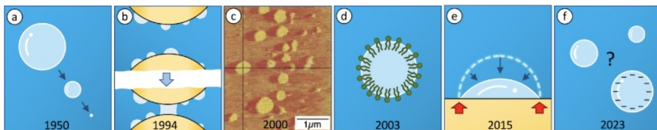
Slika 1: Zgodovinski pregled ključnih spoznanj o nanomehurčkih. (a) Konvencionalna teorija Epsteina in Plesseta pravi, da bi se morali nanomehurčki hipoma raztopiti. (b) Meritve privlačnih sil dolgega dosega, izmerjene med hidrofobnimi površinami, vodijo do hipoteze o dolgoživih nanomehurčkih na površinah. Ko se površini približata, se mehurčki zlijejo v zračni tunel, ki vleče površini skupaj. (c) Prve slike nanomehurčkov, narejene z mikroskopom na atomsko silo. [Z dovoljenjem povzeto iz Ishida idr. ( https://doi.org/10.1021/la000219r ) Avtorske pravice 2000 American Chemical Society.] (d) Prva uporaba majhnih lipidno odetih mehurčkov kot ultrazvočno kontrastno sredstvo. (e) Pripenjanje kontaktne linije razloži trajne in dolgožive nanomehurčke na površinah. (f) Prosti nanomehurčki danes ostajajo odprt problem.
