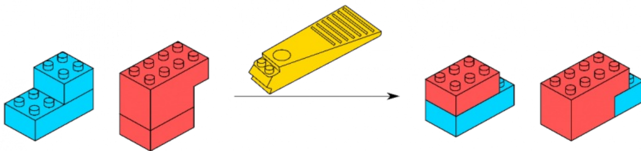
Splošna reakcijska shema za reakcije spajanja
